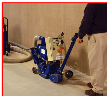
Regulacja uchwyty operatora
